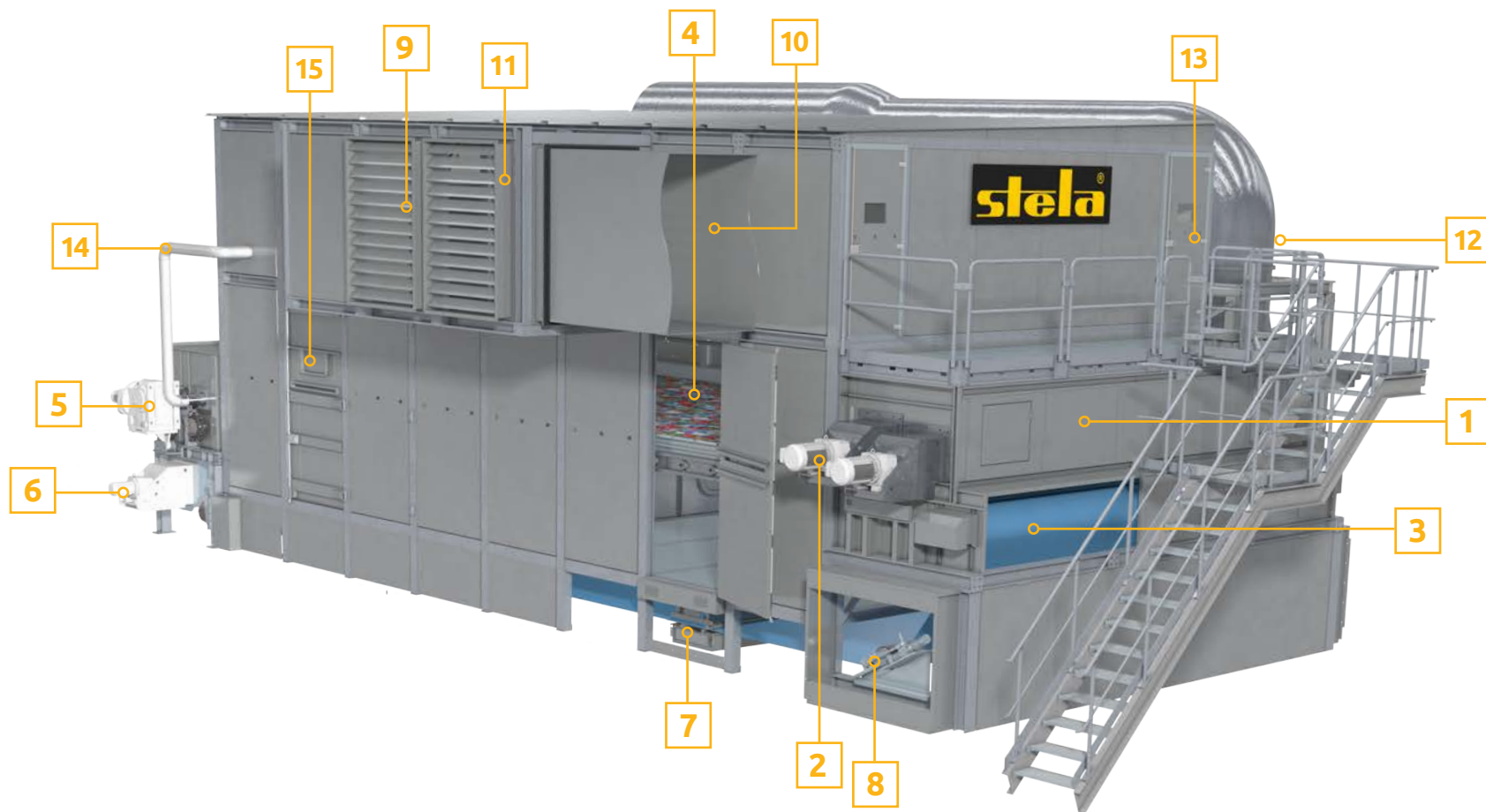
1 = 喂料端 2 = 双喂料螺旋 3 = 干燥网带 4 = 物料层 5 = 网带驱动 6 = 出料螺旋 7 = 网带水洗清洁系统 8 = 网带纠偏控制系统 9 = 新风入口 10 = 热风入口 11 = 全自动混气阀 12 = 排气风机 13 = 布风系统检修门 14 = 网带风洗清洁系统 15 = 翻料器 (可选)
